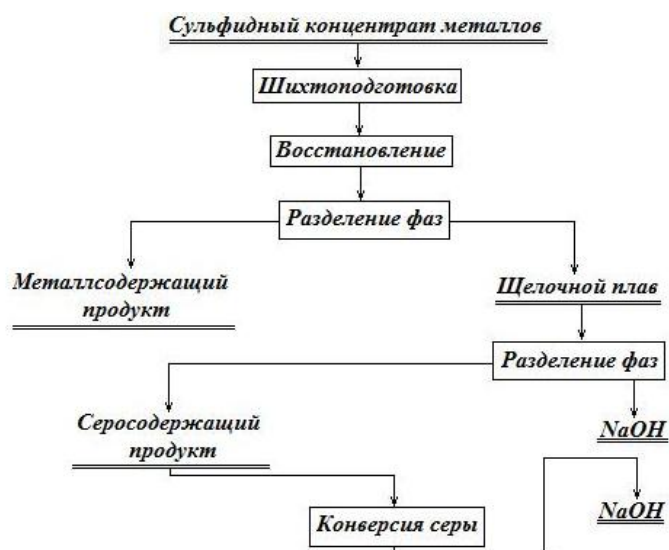
Рис. 1 Блок-схема технологического процесса восстановления металлов из сульфидных соединений
