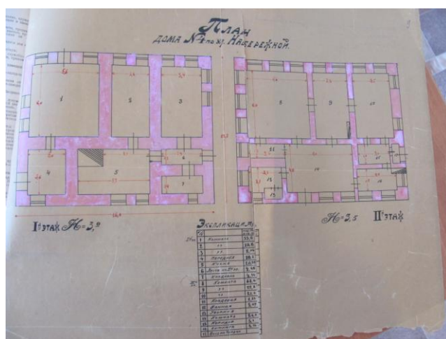
Рис.5. Планы этажей дома по ул. Набережной, 4. (из фондов МУЕА)
